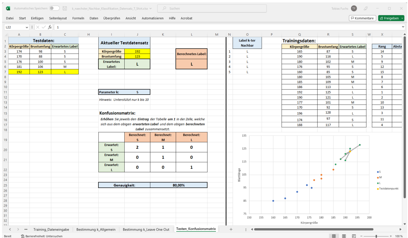
Abbildung 5: Screenshot der Tabelle zum Testen des Modells und der Ergebnisdarstellung in Form einer Konfusionsmatrix (geöffnet in Microsoft Excel)
