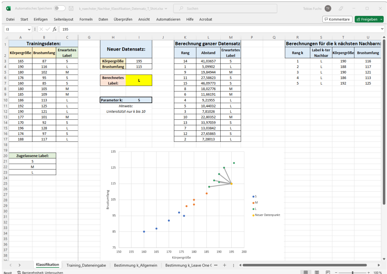
Abbildung 1: Screenshot der Tabelle zur Klassifikation eines neuen Datenpunkts (geöffnet in Microsoft Excel).
